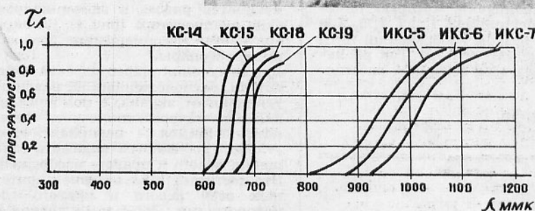
Рис. 4. Спектральная характеристика пропускания красных и черных инфракрасных стеклянных светофильтров
